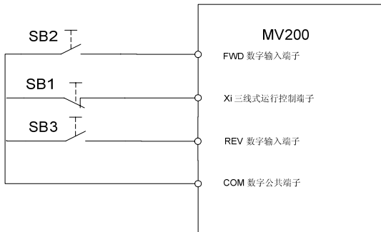
图6-20 三线式运转模式 1
