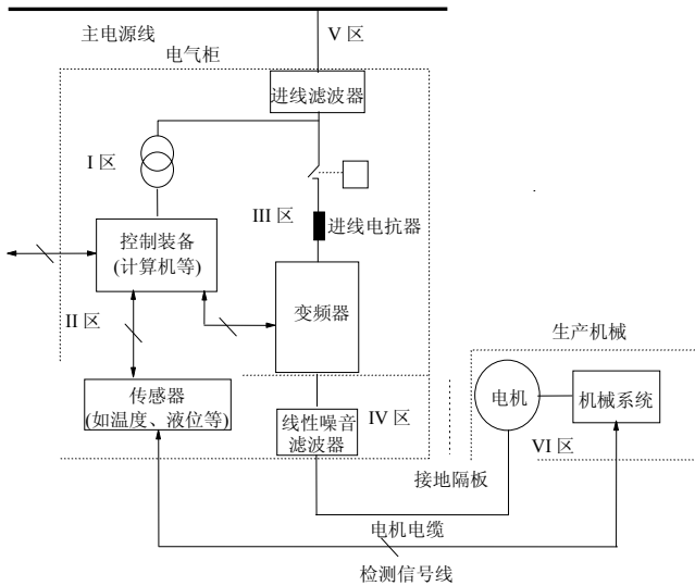
图3-33 变频器 EMC 安装推荐区域划分示意图
