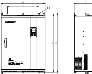
图1-4 R9~R10 箱体产品外形和安装尺寸示意图
