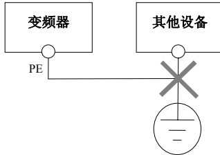
图3-29 接地示意图 3
