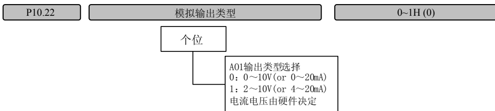
图6-40 模拟输出类型选择
