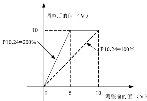
图6-41 模拟输出与增益关系曲线
