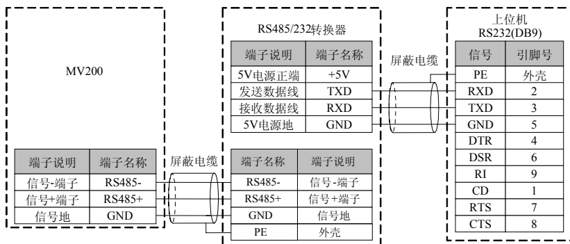
图3-9 RS485-(RS485/232)-RS232 通讯配线
