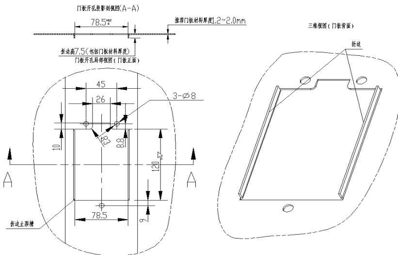
图1-9 操作面板固定座安装孔尺寸
