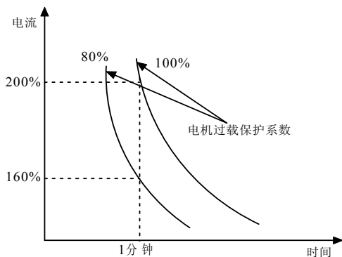
图6-10 电机过载保护系数设定
