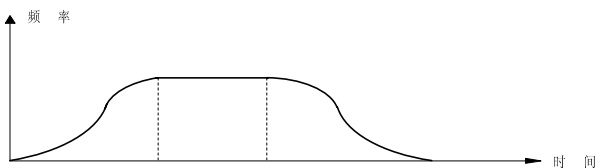
图6-44 S 曲线加减速
