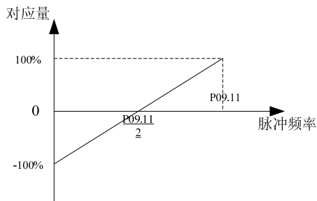
图6-24 中心点模式 2
