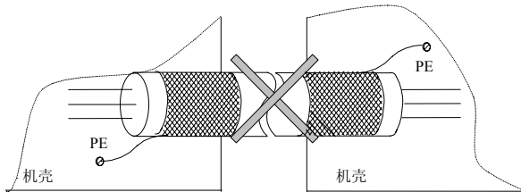
图3-26 错误的屏蔽接地方法
