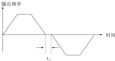
图6-17 正反转死区时间
