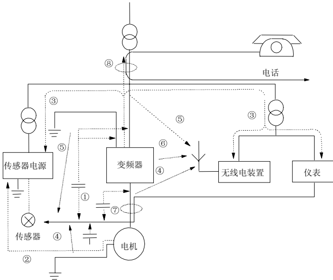
图3-23 噪声传播路径示意图
