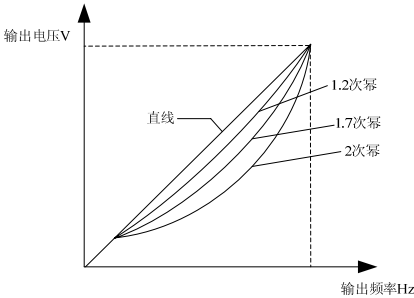
图6-13 V/F 曲线
