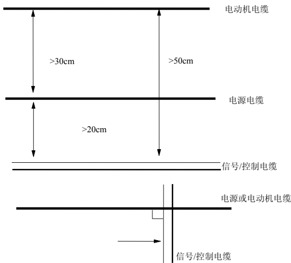
图3-24 系统配线要求
