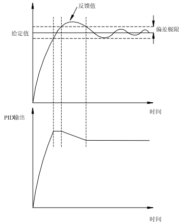
图6-60 偏差极限示意图
