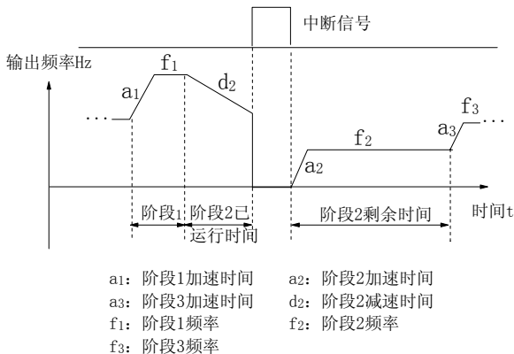
图6-56 PLC 起动方式 1
