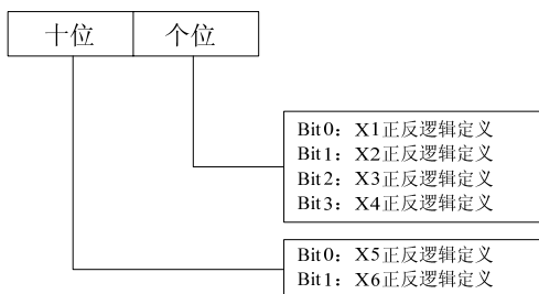
图6-25 端子正反逻辑设定
