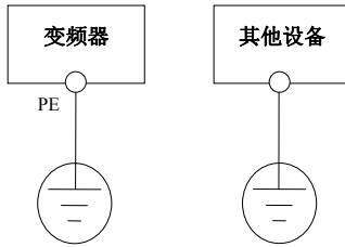
图3-27 接地示意图 1
