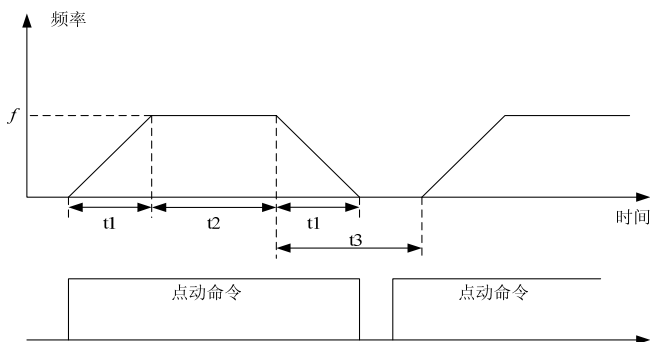
图6-48 点动运行参数说明
