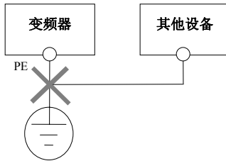
图3-30 接地示意图 4
