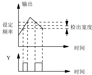
图6-27 频率到达信号输出示意图
