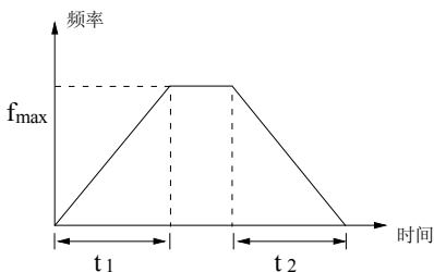
图6-43 直线加减速
