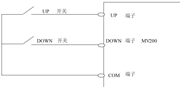
图6-6 数字设定 2 方式时接线示意图
