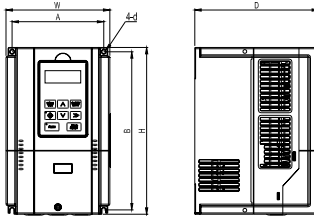
图1-2 R3~R4 箱体产品外形和安装尺寸示意图
