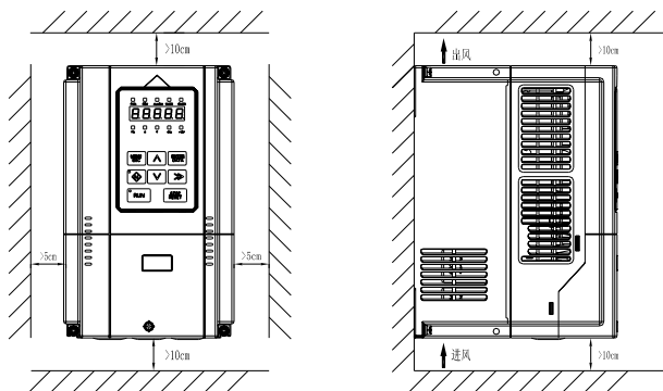
图2-2 55kW G/55kW P 及以下产品安装间隔距离
