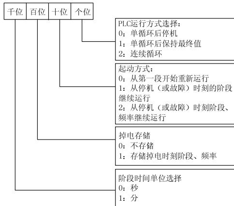
图6-52 简易 PLC 运行方式选择
