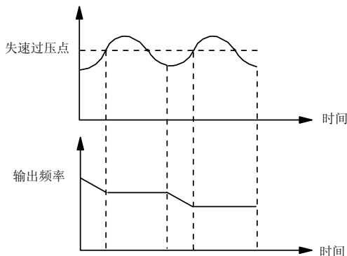
图6-71 过压失速功能
