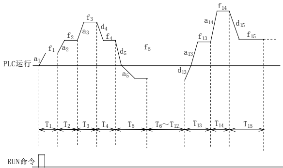
图6-54 PLC 单循环后保持方式
