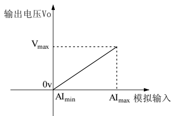
图6-37 输出电压曲线
