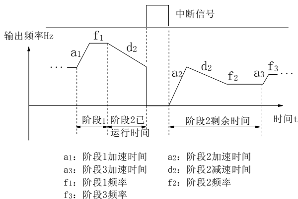
图6-57 PLC 起动方式 2
