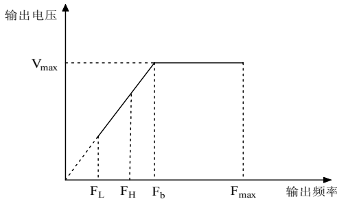
图6-8 极限频率参数定义示意图
