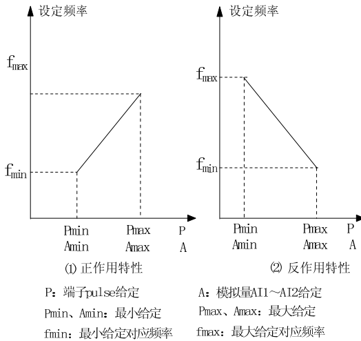
图6-33 模拟输出频率特性曲线
