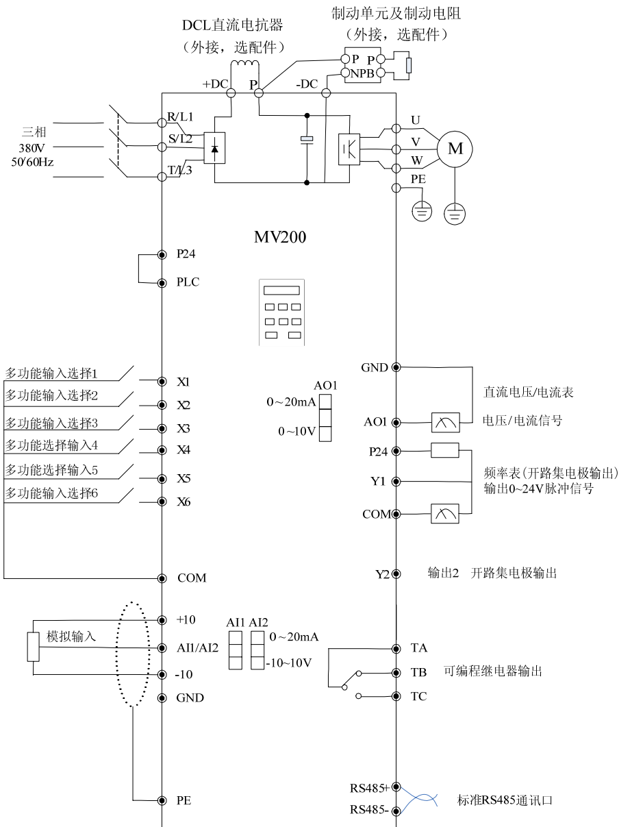
图3-4 基本配线图 2
