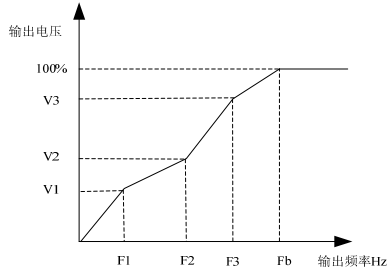
图6-14 多段 V/F 曲线
