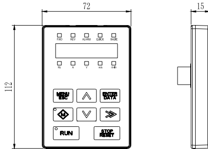
图1-7 操作面板的外形和安装尺寸
