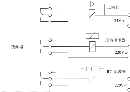
图3-31 继电器、接触器及电磁制动器要求
