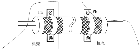
图3-25 正确的屏蔽接地方法
