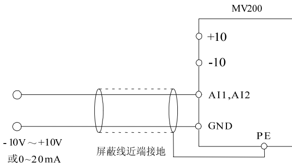
图3-6 AI1、AI2 端子端子配线图
