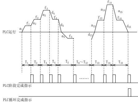
图6-51 简易 PLC 运行图
