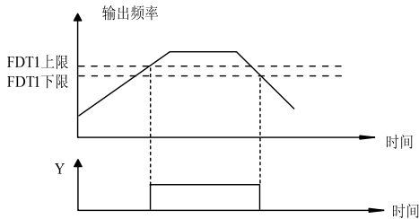
图6-28 频率水平检测示意图
