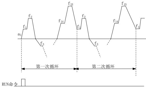
图6-55 PLC 连续循环方式
