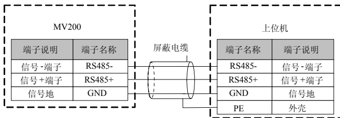
图3-8 RS485-RS485 通讯配线
