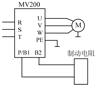
图附 2-1 变频器与制动电阻连接图
