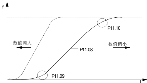
图6-46 S 曲线调整示意图说明
