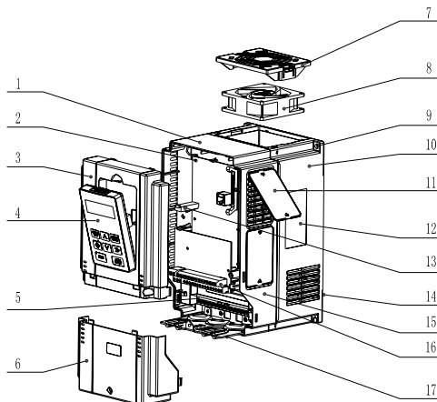
1.中壳 2.主控板 3.上盖板 4.操作面板 5.主回路接线端子 6.下盖板 7.风扇卡罩 8.风扇
