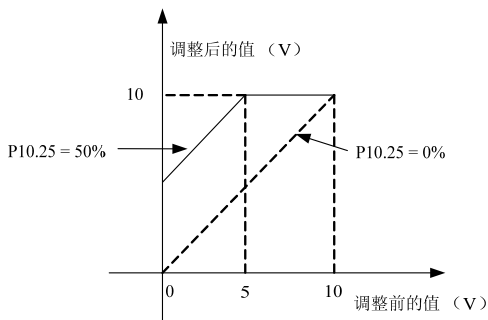
图6-42 模拟输出与零偏关系曲线
