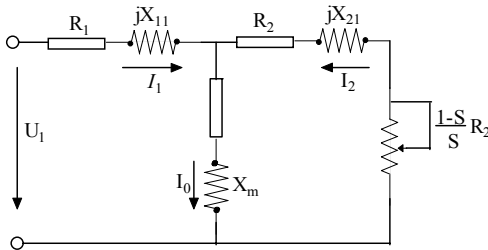
图6-9 异步电机稳态等效电路图
