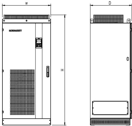
图1-5 R11 箱体产品外形和安装尺寸示意图
