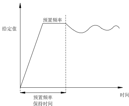
图6-61 PID 预置频率运行示意图
