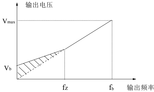
图6-15 转矩提升（提升量为阴影部分）
