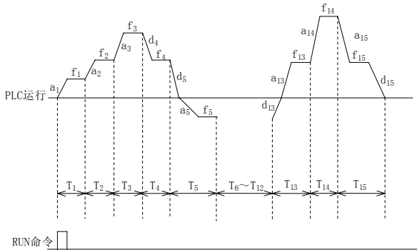
图6-53 PLC 单循环后停机方式
