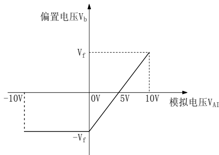
图6-36 输出电压偏置
