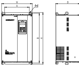
图1-3 R5~R8 箱体产品外形和安装尺寸示意图
