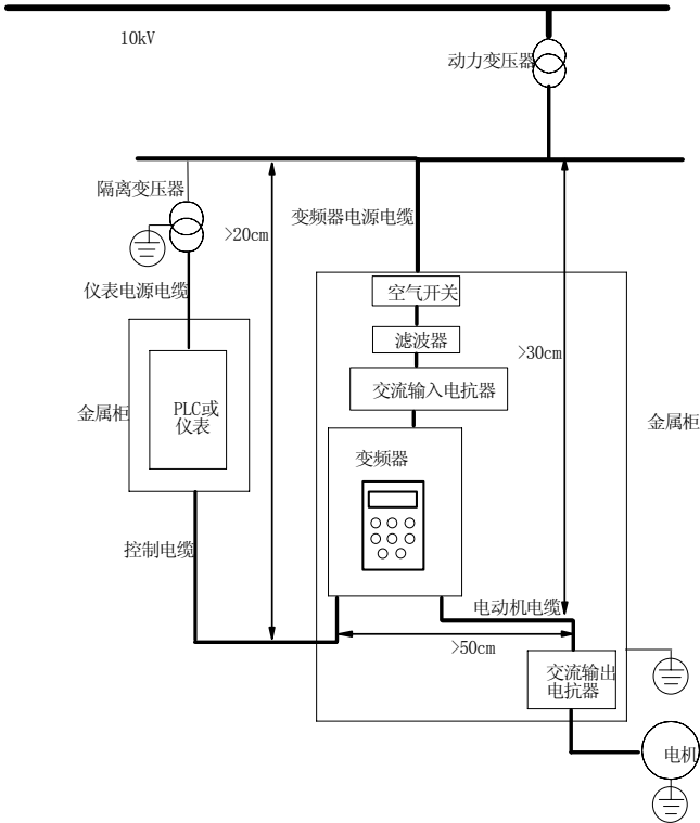
图3-34 变频器的安装示意图
