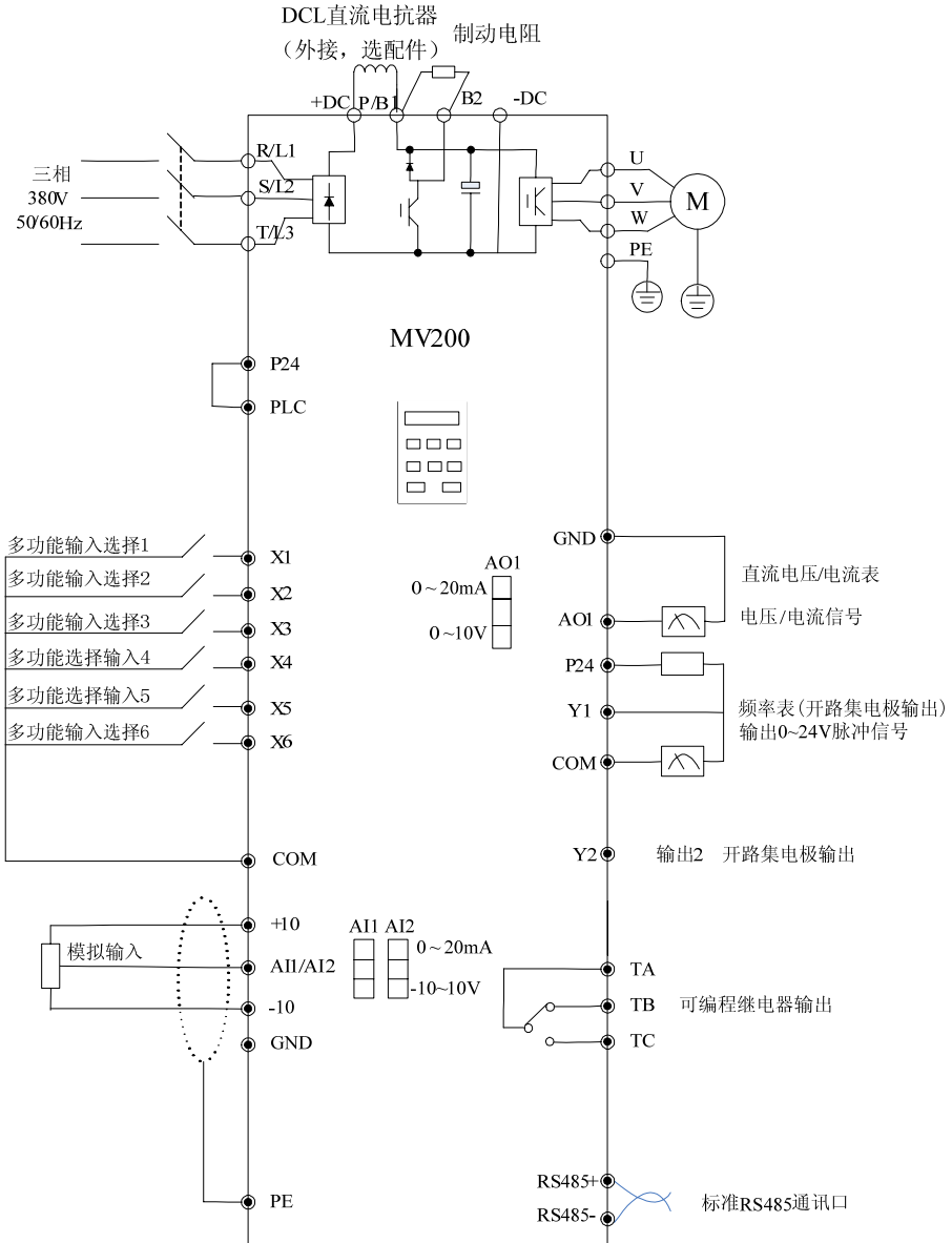
图3-3 基本配线图 1
