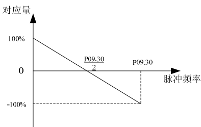
图6-30 中心点模式 1
