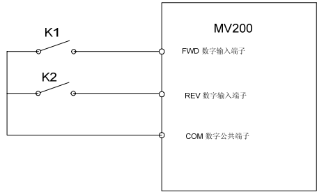
图6-19 两线式运转模式 2
