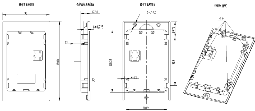
图1-8 操作面板固定座外形尺寸
