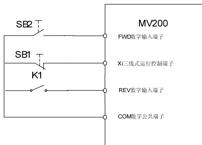
图6-21 三线式运转模式 2
