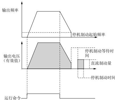
图6-16 减速停车+直流制动示意图
