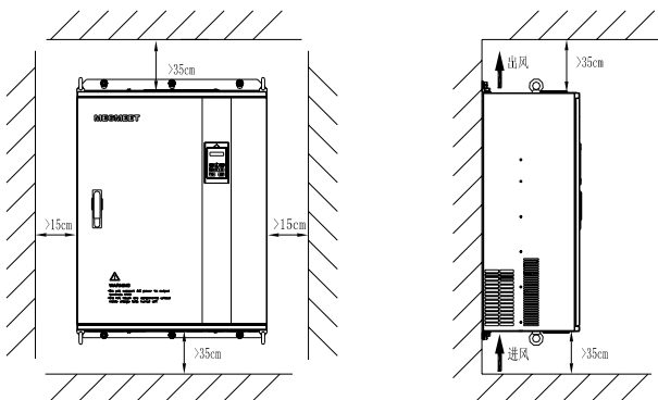
图2-3 75kW G/75kW P 及以上产品安装间隔距离
