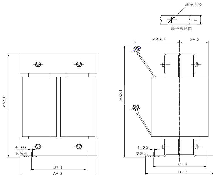
图1-6 直流电抗器的外形图
