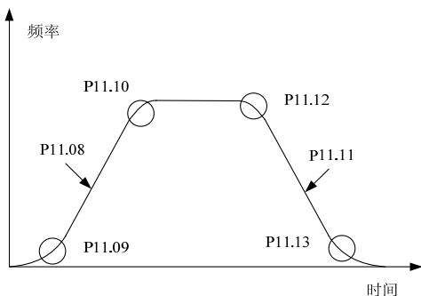
图6-45 S 曲线参数示意图
