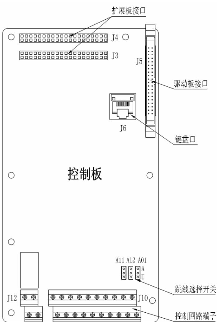
图3-21 控制板示意图
