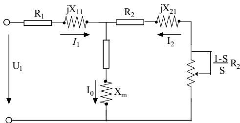
图6-11 异步电机稳态等效电路图
