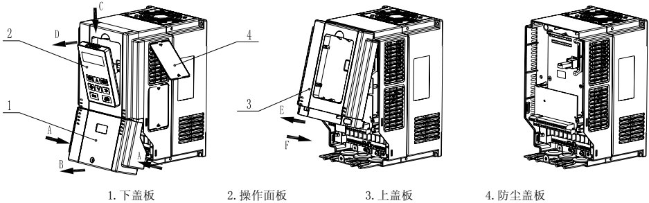
图2-1 变频器部件的拆卸安装示意图（以 R4 为例）
