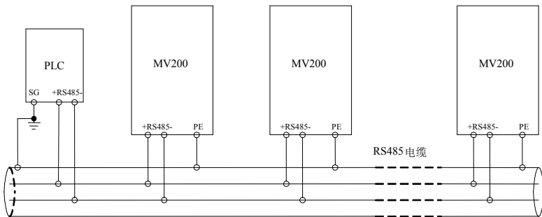
图3-10 PLC与变频器多机通讯时推荐的接线图（变频器、电机全部良好接地）
