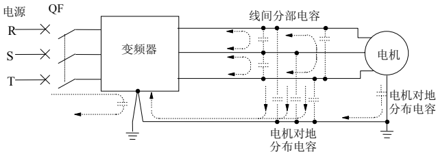
图3-32 漏电流路径
