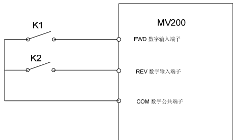
图6-18 两线式运转模式 1
