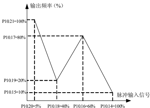
图6-39 脉冲信号输入实例参数设置
