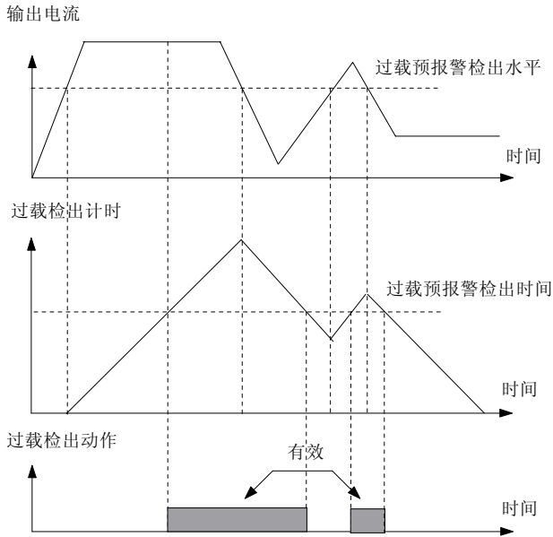
图6-70 过载预警检出功能示意图
