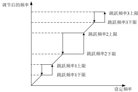
图6-49 跳跃频率及范围示意图
