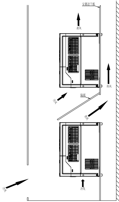
图2-4 两台变频器以上的安装
