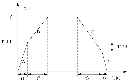
图6-47 加减速时间 1、2 切换示意图
